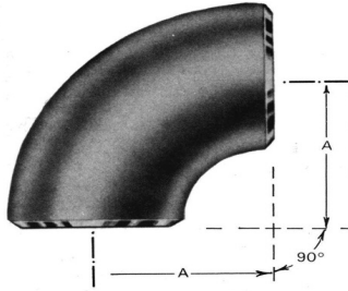
90° long radius Elbow
